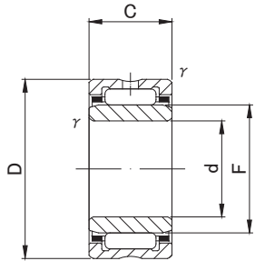
NA49,NA59,NA48,NKI
