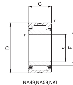
NA49,NA59,NKI
