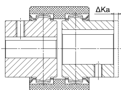
Odchyłka osiowa
