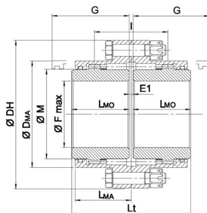
Wykonanie A
