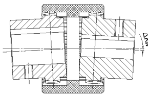
Odchyłka kątowa
