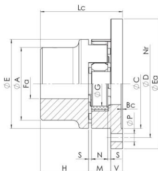
Kołnierz - wał
