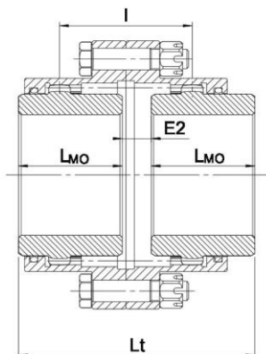
Wykonanie B
