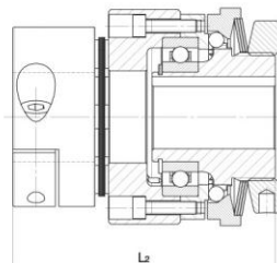
Wykonanie z otworem i rowkiem wpustowym / GSM
