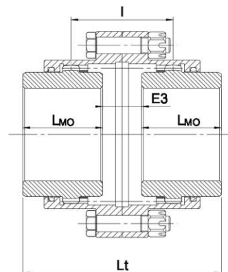
Wykonanie C
