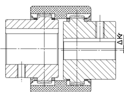
Odchyłka promieniowa
