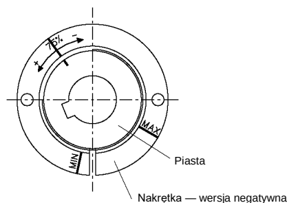
Nakrętka — wersja negatywna
