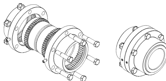
Wykonanie specjalne z wałem pośrednim
