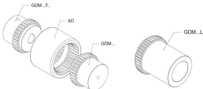
Sprzęgła standardowe
