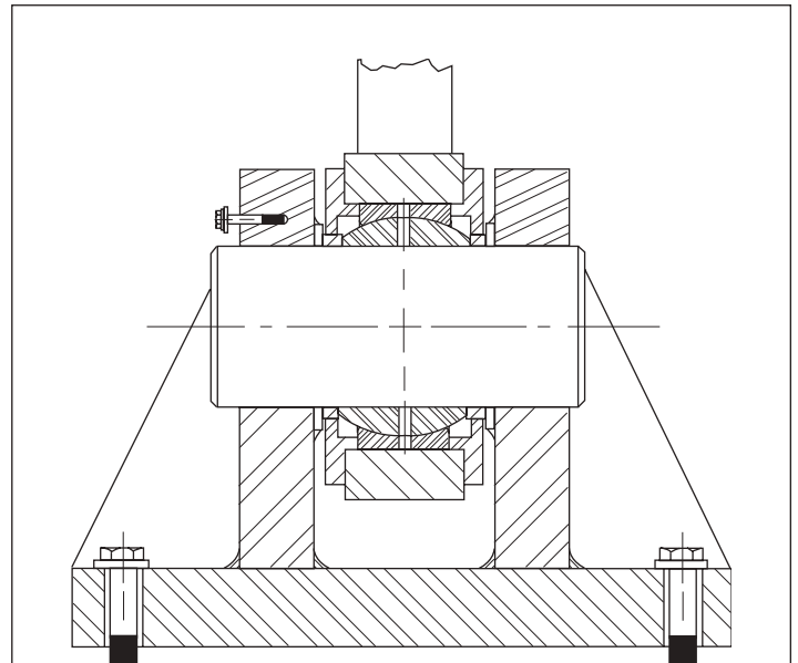
Hinge Pin
